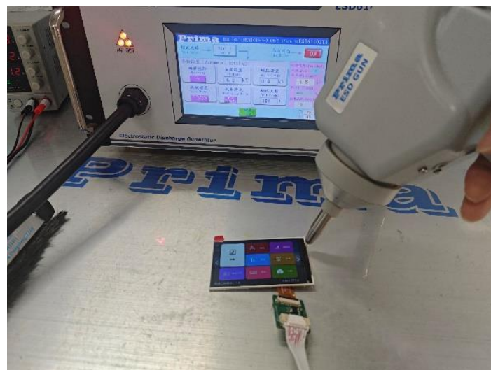
图 5-2 ESD 测试图
