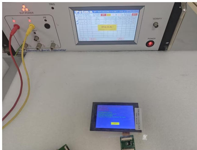
图 5-3 EFT 测试图
