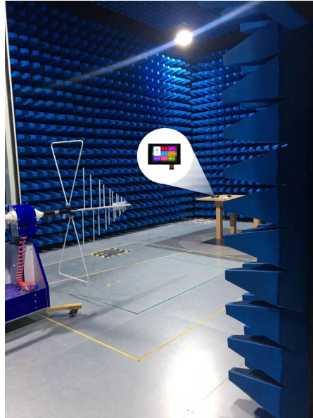
图 5-5 RE 测试图
