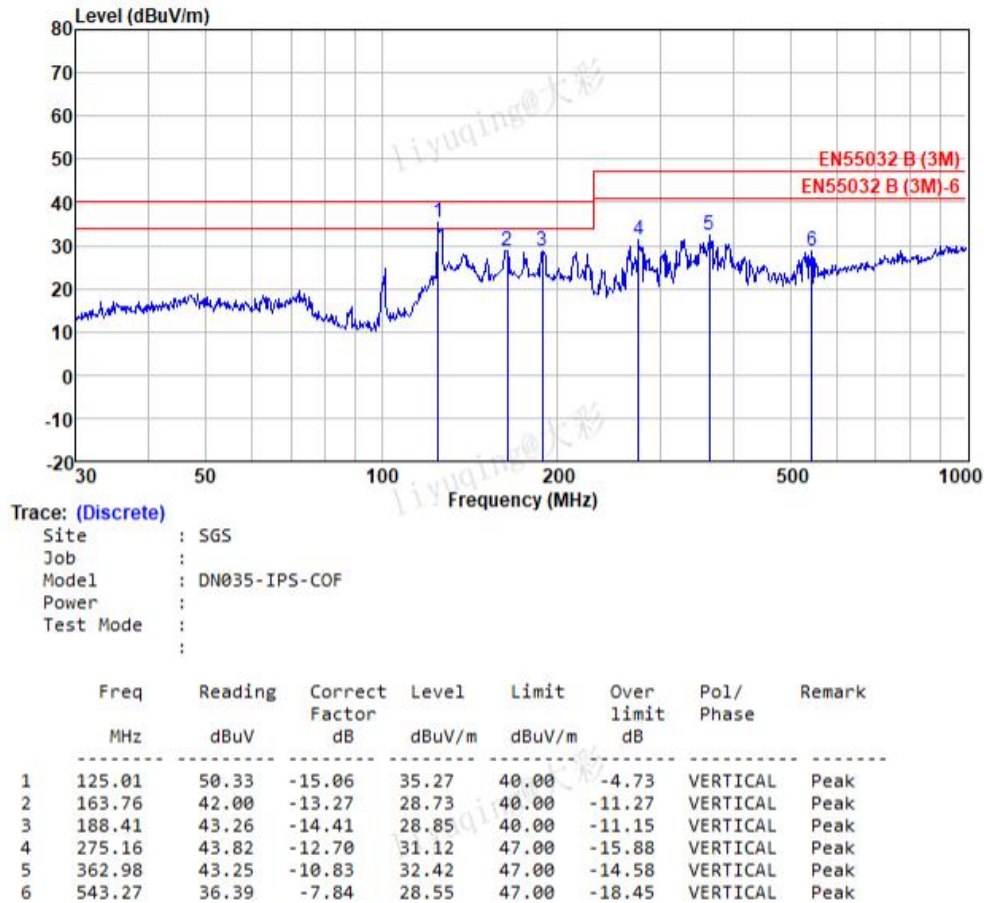
图 5-7 RE 测试垂直方向
