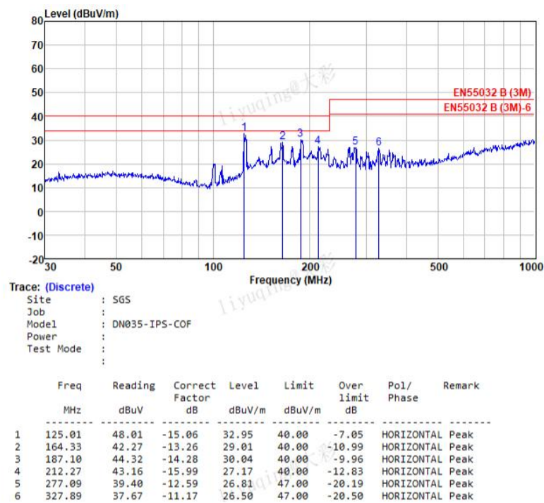
图 5-6 RE 测试水平方向
