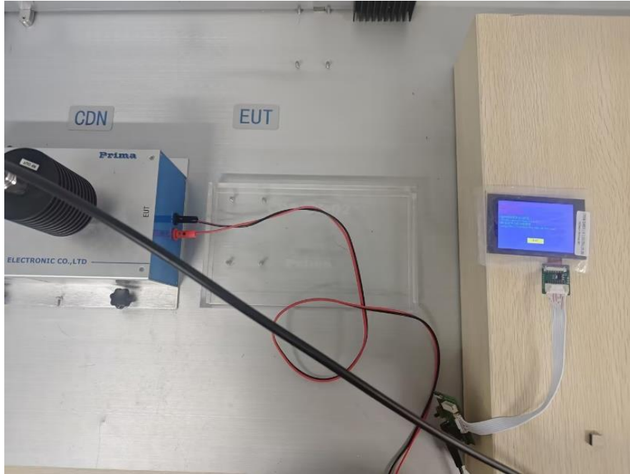
图 5-4 传导抗扰度测试图
